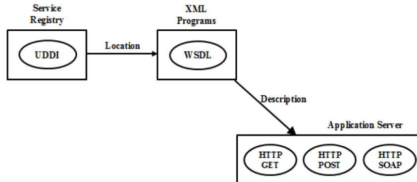
Gambar 3.5 Kombinasi UDDI, SOAP, dan WSDL untuk pembentukan registry (Cheng, 2008)
