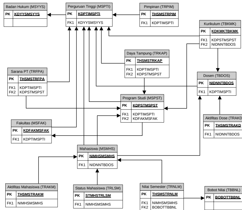
Gambar 5.4. Relasi tabel
