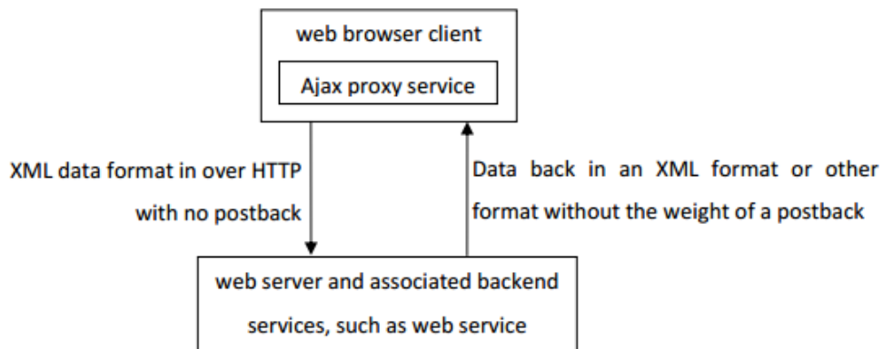
Gambar 3.6 Ajax
