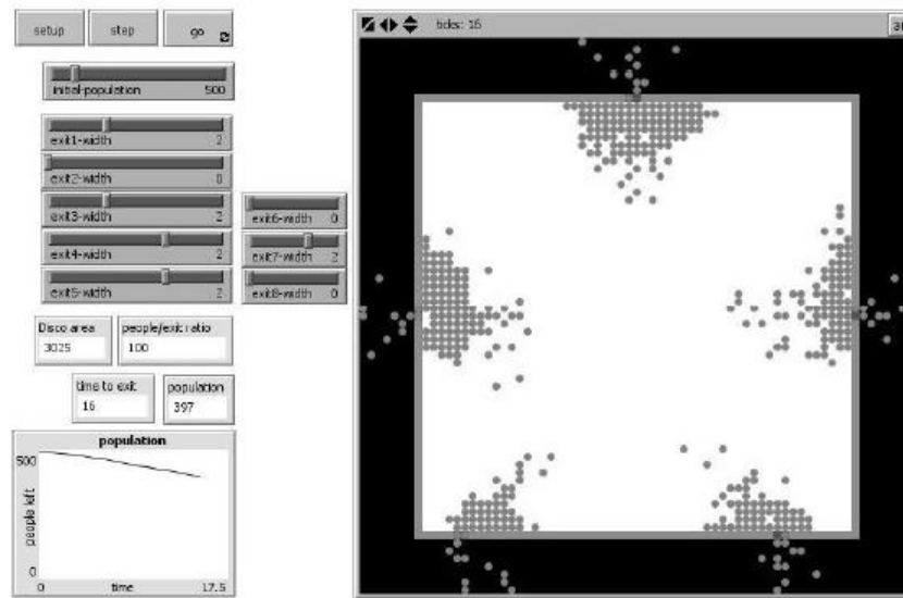
Gambar 2.2. Simulasi Menggunakan NetLogo (Almeida dkk., 2010)
