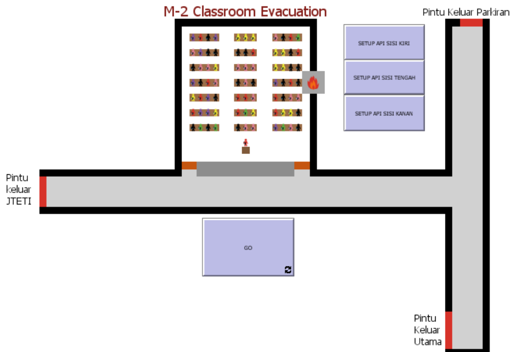
Gambar 5.24 Pemodelan Skenario Pelebaran Pintu Ruang M-2
